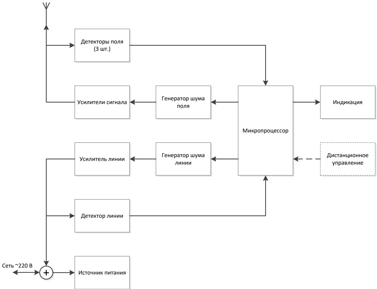
Рисунок 1 – Функциональная схема
